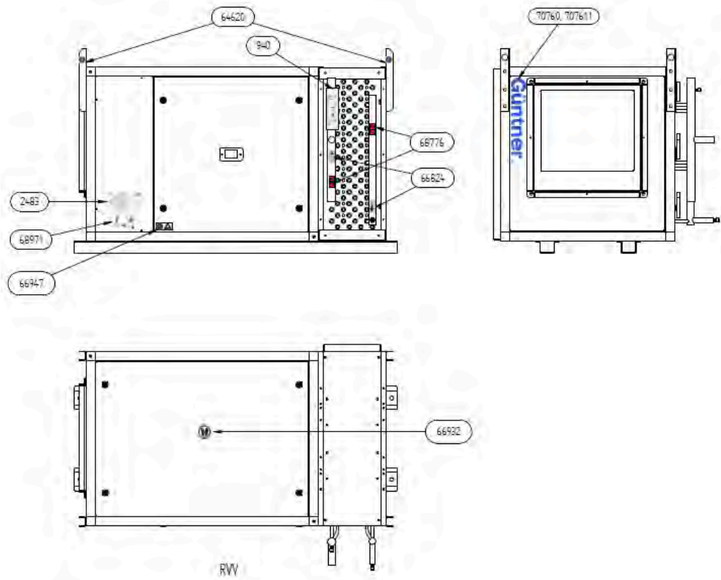
Kennzeichnungen am RVV
