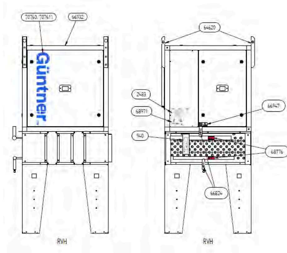
Kennzeichnungen am RVH
